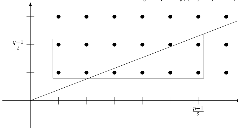
Obr. 4.2: Ilustrácia dôkazu zákona kvadratickej reciprocity, prípad p = 13, q = 5
